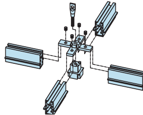
Type BK
