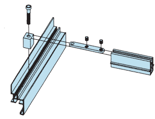
Type WB 1
